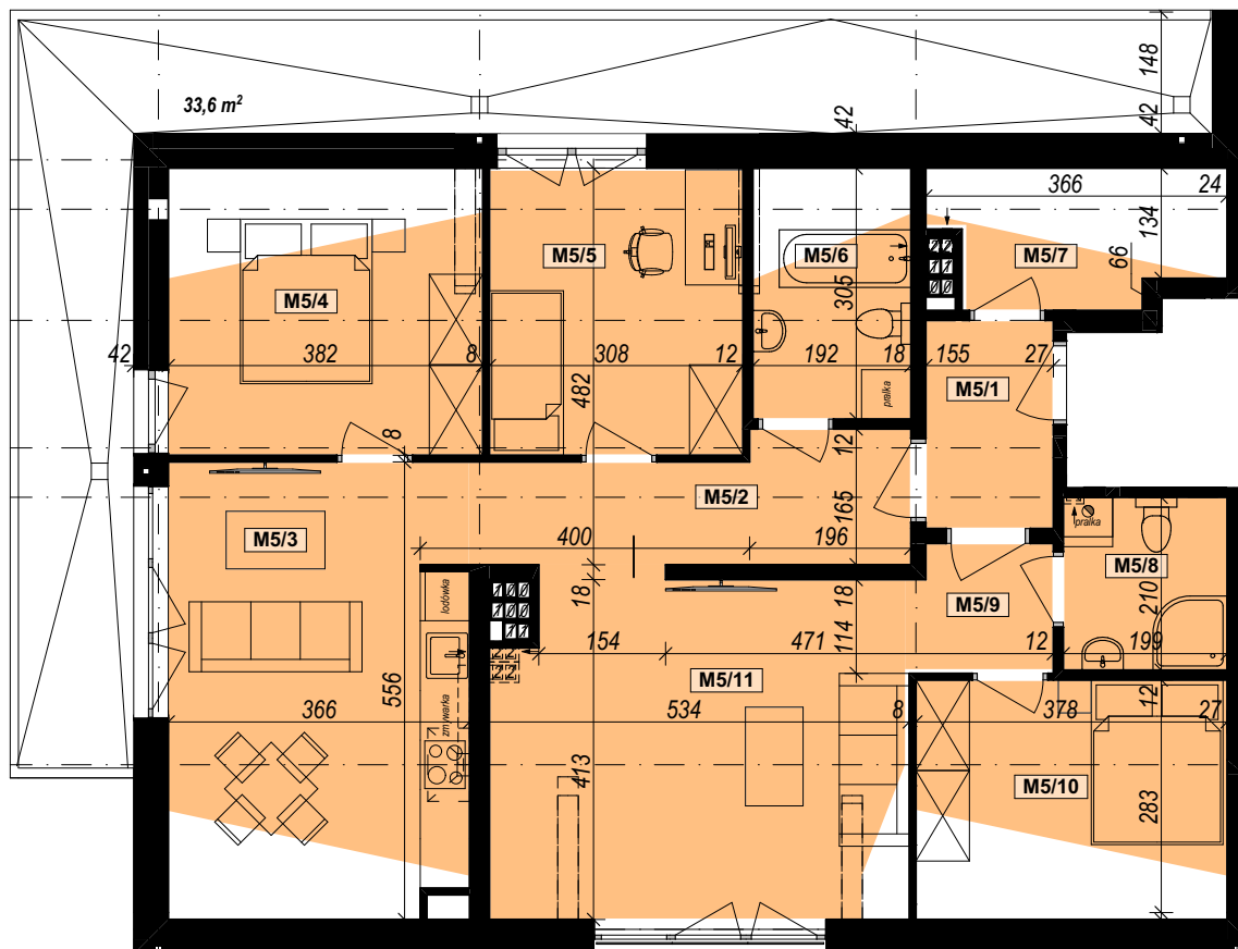
RZUT MIESZKANIA
