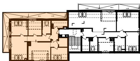
SCHEMAT KONDYGNACJI
